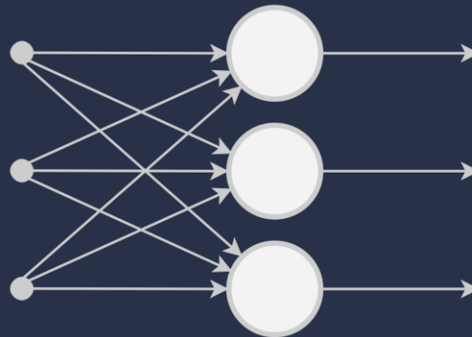
Yolact Netzwerk
